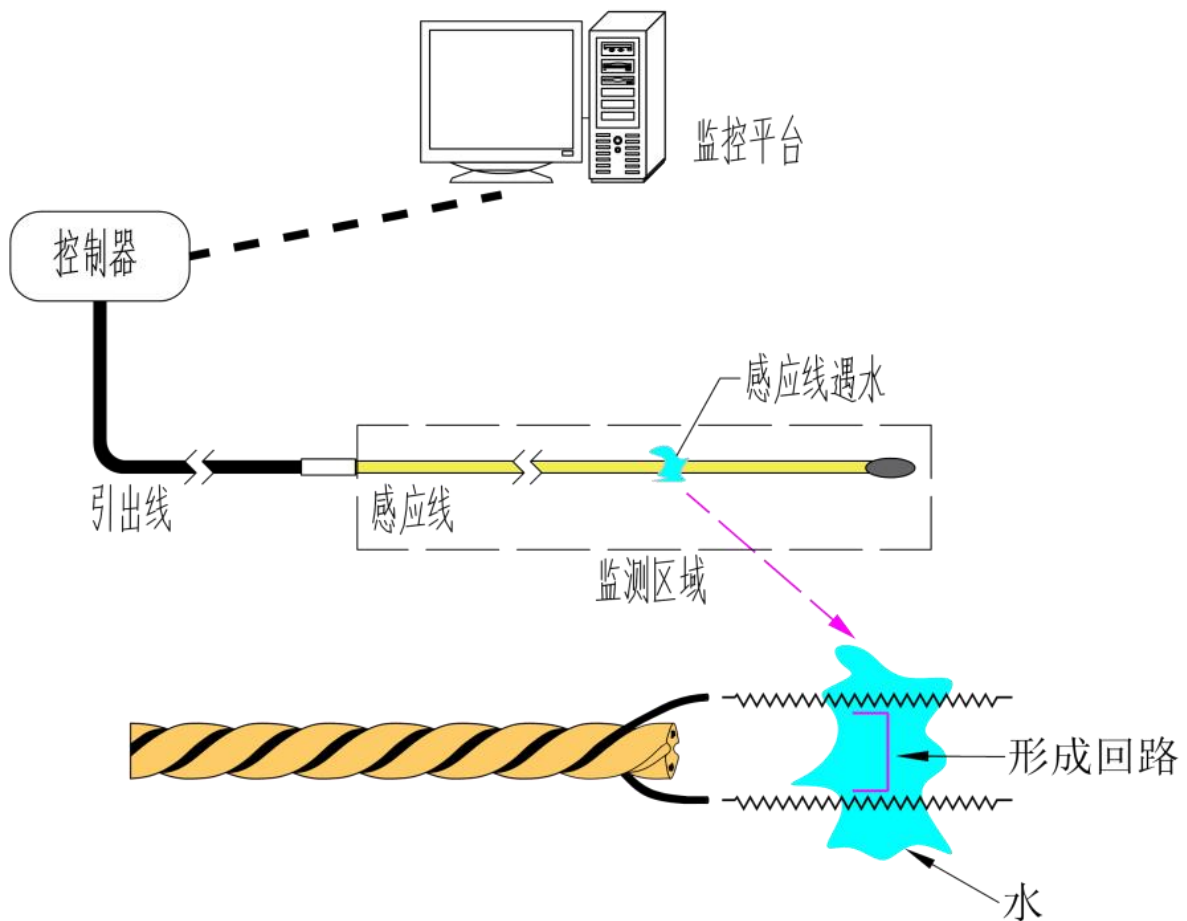
图 1 原理示意图
